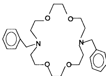
dibenzylodiaza 18C6
