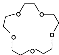
15C5
