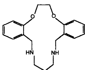
dibenzodiaza 15C4
